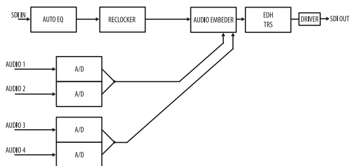
Blok šema DVA-12e
