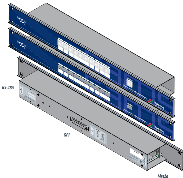
NSCU-10S - daljinska komanda sa malim tasterima za 10x1 svičere, prednji panel
